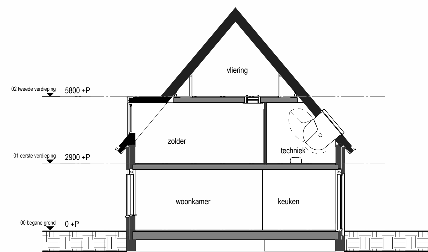
Doorsnede
