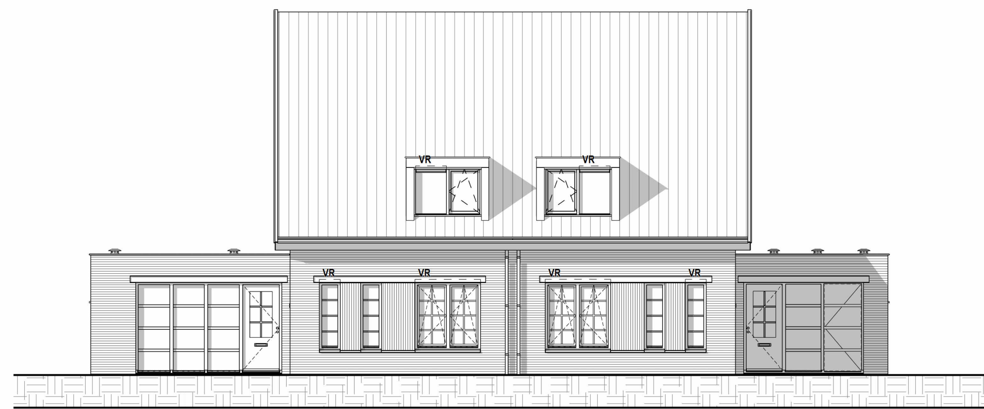
Voorgevelaanzicht
